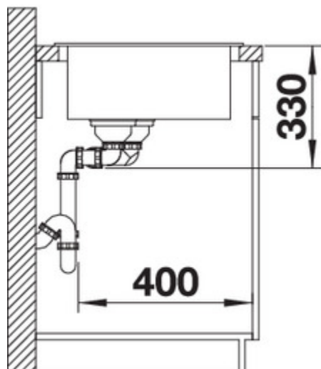
Vue latérale
